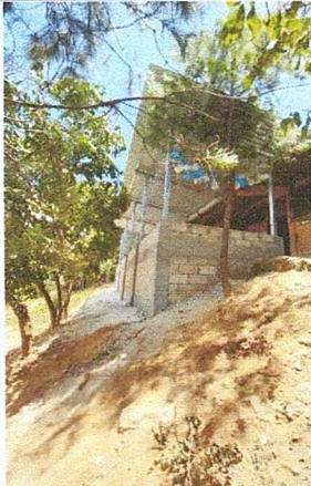
Foto 3: Area donde se realizó Mejoramiento de muro de contención, mejoramiento de muro perimetral, Mejoramiento con estructura tipo portico y lámina troquelada calibre 26 y Mejoramiento de losa de piso.
