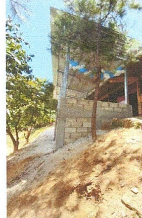
Foto 4: Area donde se realizó Mejoramiento de muro de contención, mejoramiento de muro perimetral, Mejoramiento con estructura tipo portico y lámina troquelada calibre 26 y Mejoramiento de losa de piso.
